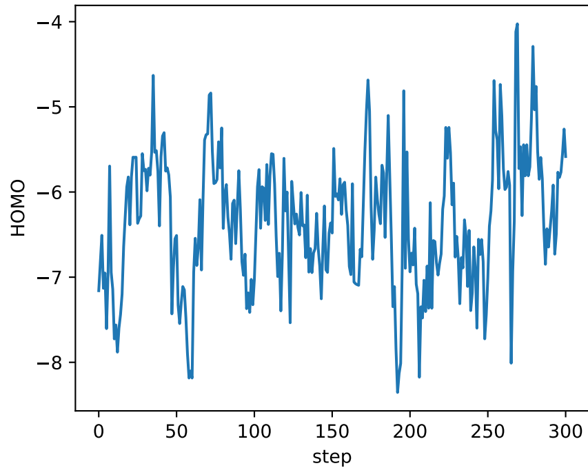
HOMO - evolution
