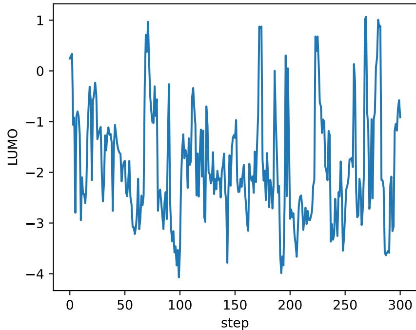
LUMO - evolution
